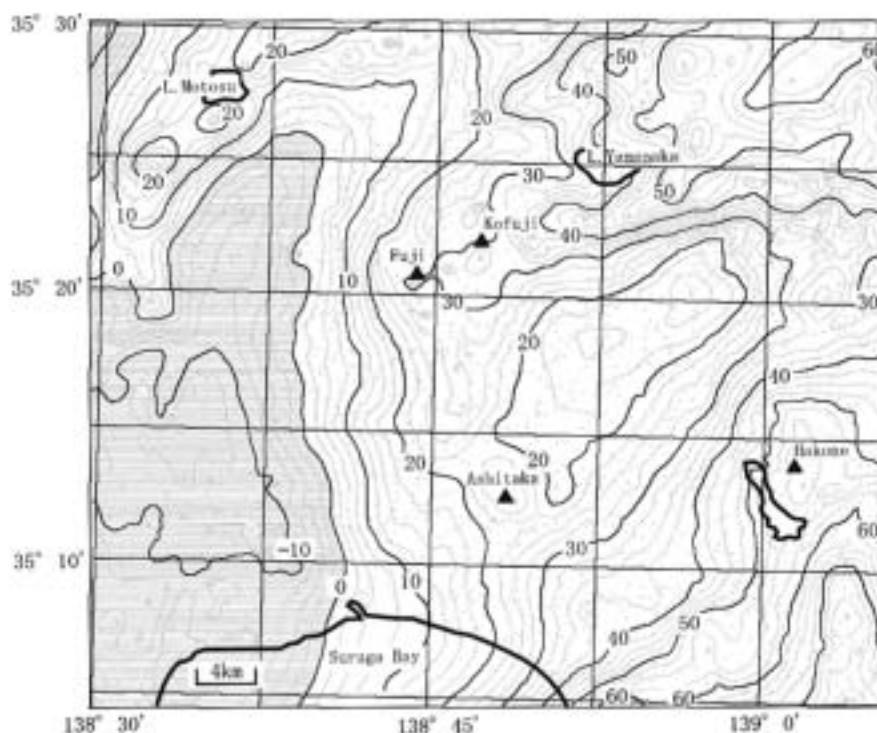
図13 富士山周辺のブーゲー異常図(駒澤 2000)。密度は 2.3 \text{ g/cm}^3 を仮定。単位は mGal。
